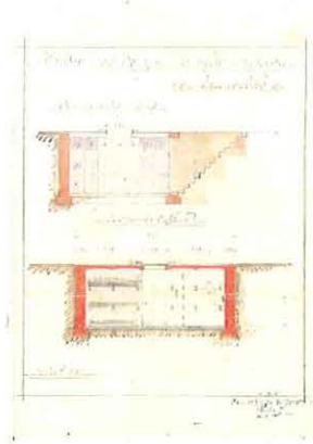
Foto 10: ontwerpplan 1921
