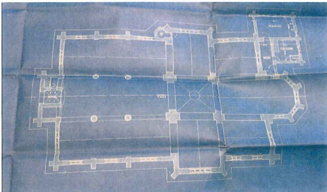
Ontwerp voor het herbouwen van de kerk, Theo Raison, 1921. Een ruime sacristie aan de zuidoostzijde wordt later aan het plan toegevoegd (Bron: Decanaal archief Diksmuide, Vladslo, nr. 1)
