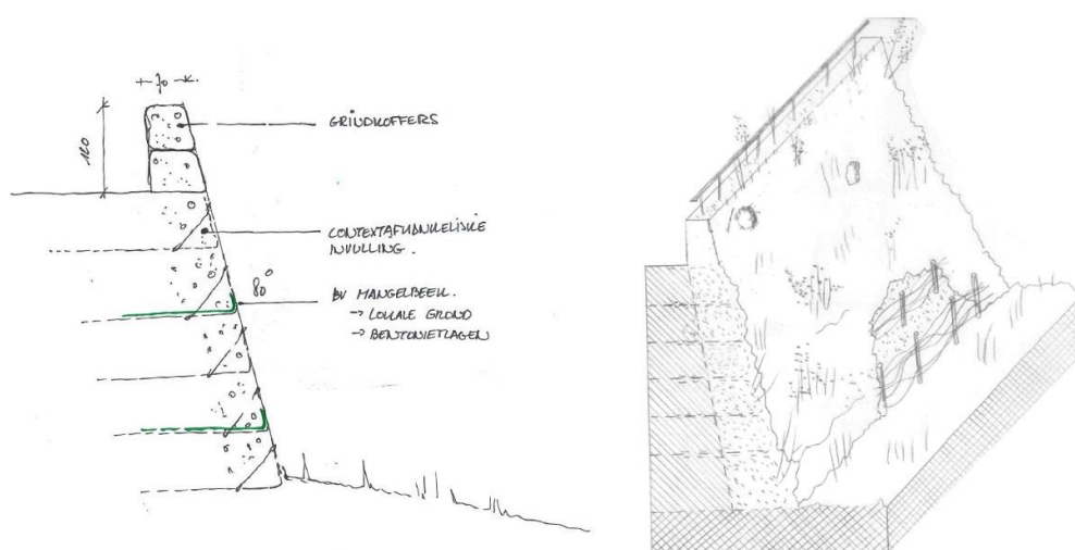
Figuur 11 - Principe ontwerp van de levende muur
