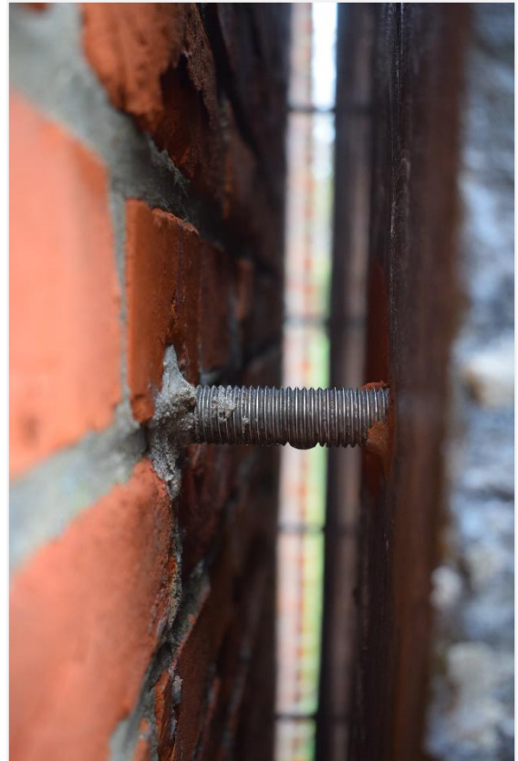
Foto 11: Heropgerichte gedenksteen. Detail verankeringssysteem
