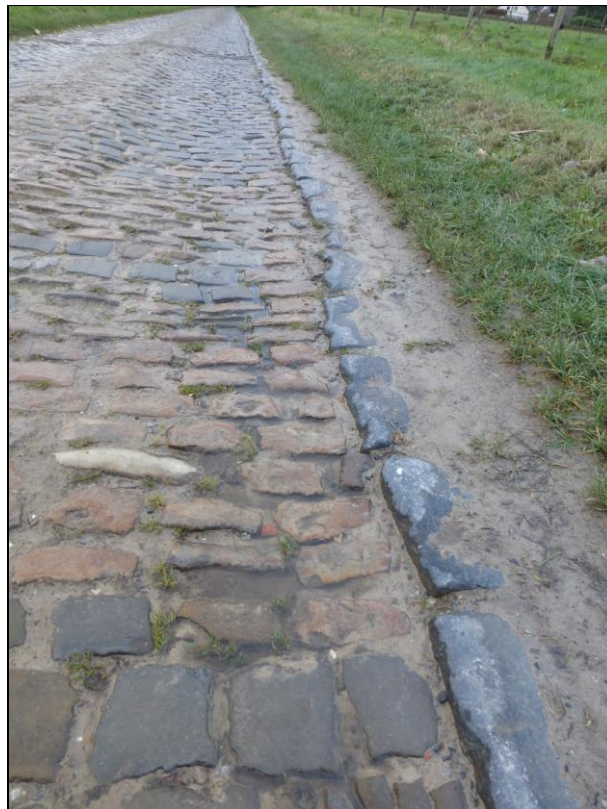
Foto 7: lichte spoorvorming.
