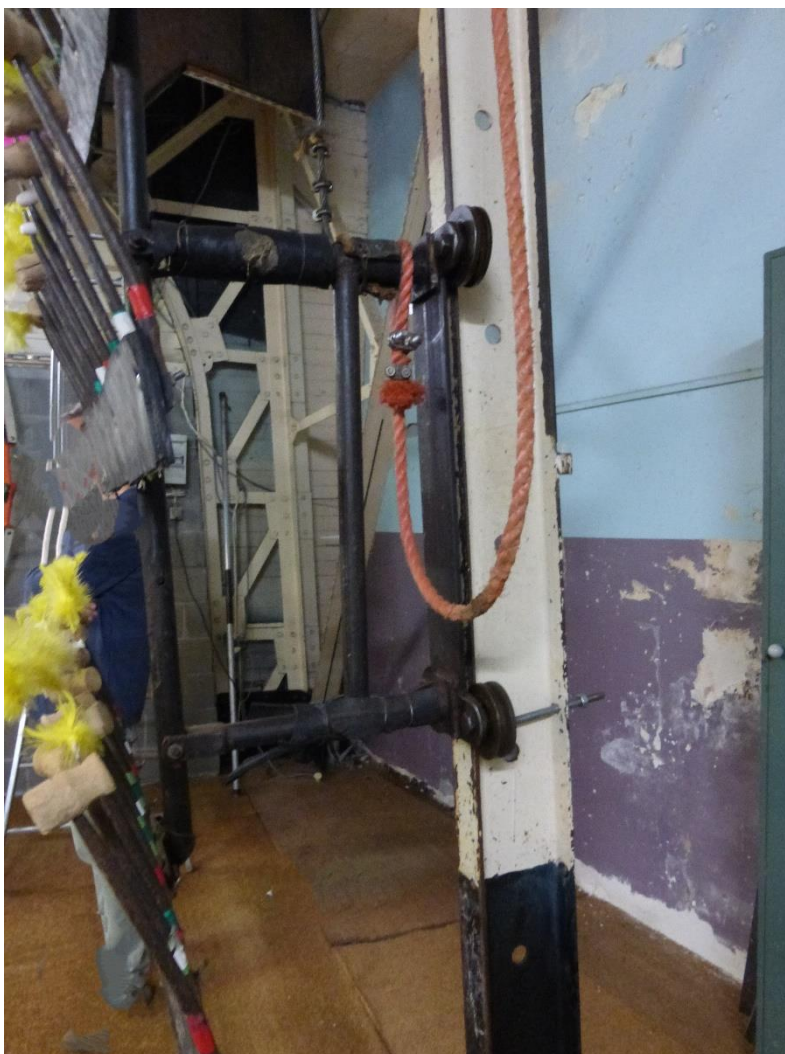
Foto 31: de oostelijke, metalen staande wip met schuifstelsysteem met wieltjes en touw voor de metalen prang (plaatsbezoek Onroerend Erfgoed 16.05.2022).
