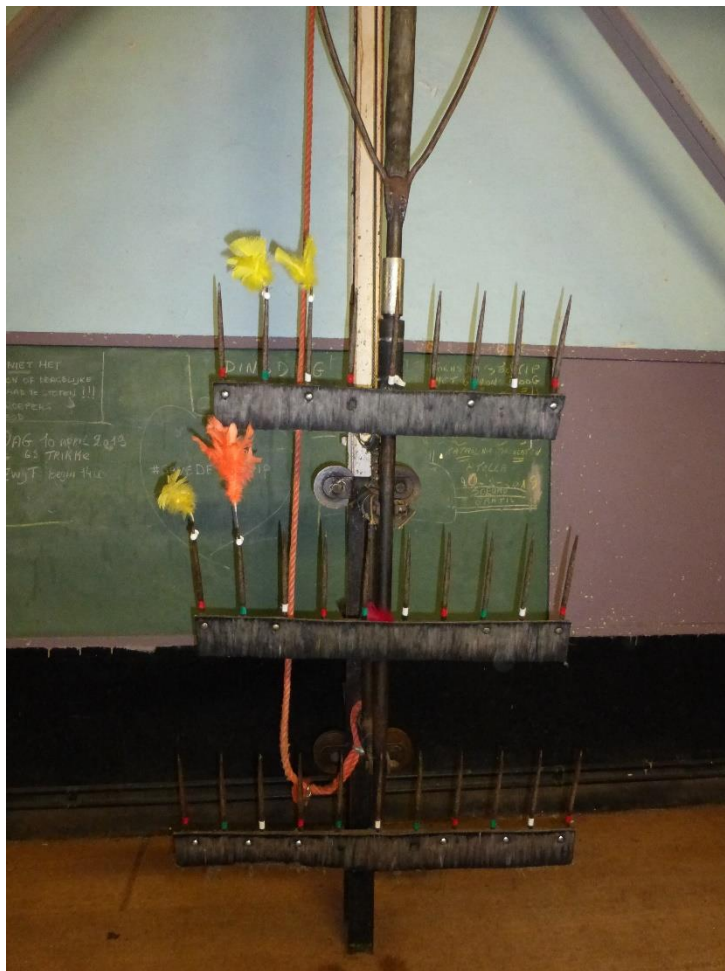
Foto 29: de westelijke, metalen staande wip met daarop de metalen prang met "vogels" (plaatsbezoek Onroerend Erfgoed 16.05.2022).
