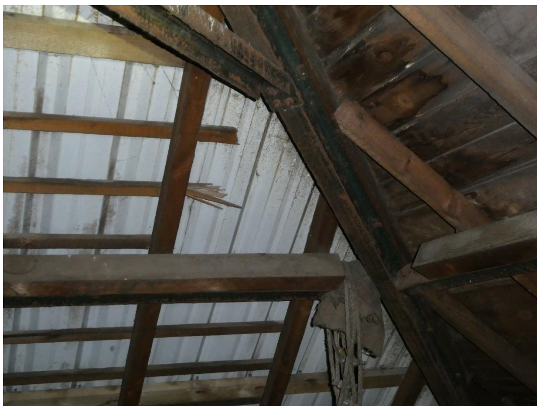
Foto 26: zolder – metalen hoekrib – deels bewaarde houten bebording (rapport Monumentenwacht, Wim Meers, plaatsbezoek 30.01.2023, © Monumentenwacht).
