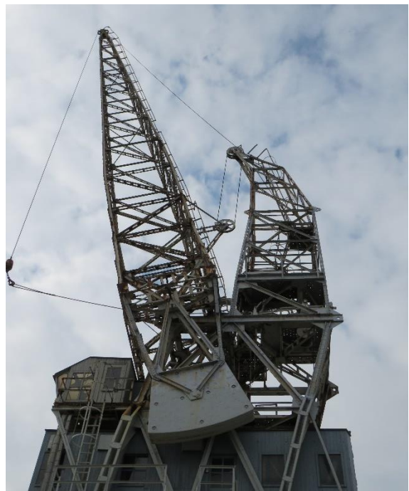
Foto 21: Zicht op giek en tegengiek (14.10.2021).
