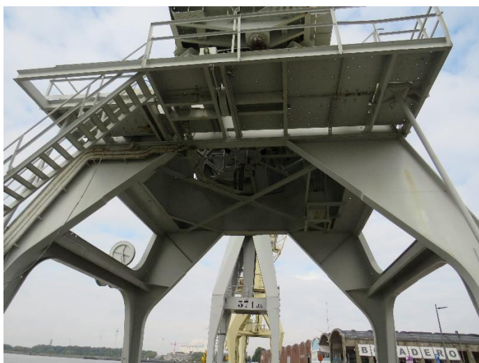
Foto 13: Portaal met bordes (14.10.2021).
