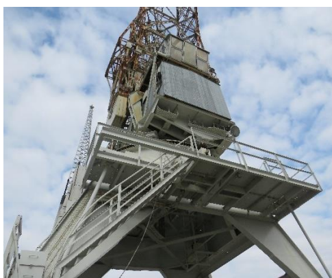
Foto 15: Bordes met bovenliggende machinekamer (14.10.202).
