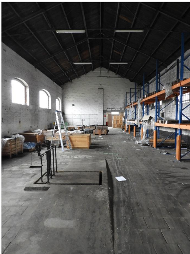
Foto 19: Fuelloods Centrale Werkplaats Mechelen. Overzicht opslagruimte gelijkvloerse verdieping deel oost (agentschap Onroerend Erfgoed 16 februari 2022)
