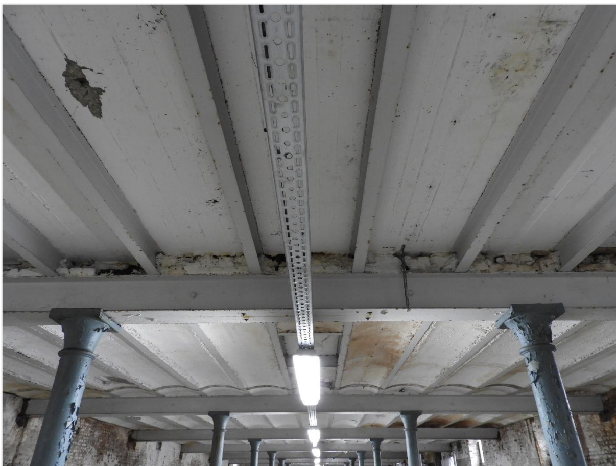
Foto 32: Fuelloods Centrale Werkplaats Mechelen. Overzicht opslagruimte kelder met deels bewaarde troggewelven (agentschap Onroerend Erfgoed 16 februari 2022)
