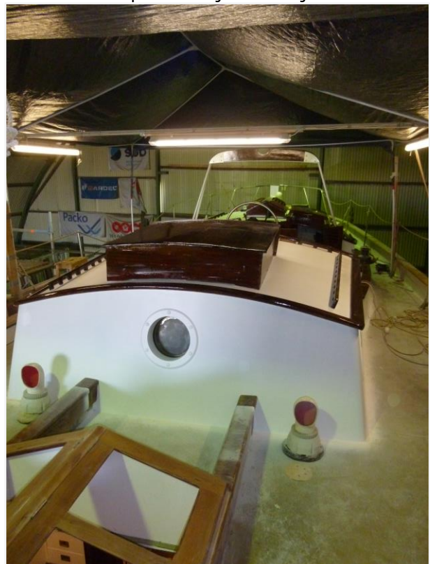
Foto 10: lichtkoepel verblijf en opbouw kajuit verblijf
