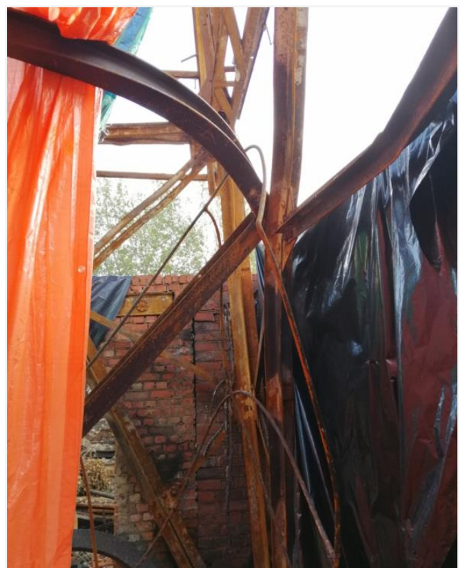
Foto 6: Vervormingen aan de het staalskelet (voet hoek noord-oost, 29 oktober 2020)
