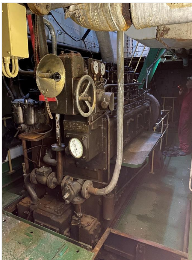
Foto 29: machinekamer met motor, schroefsnijder en draaizin bediening, koperen spreekbuis
