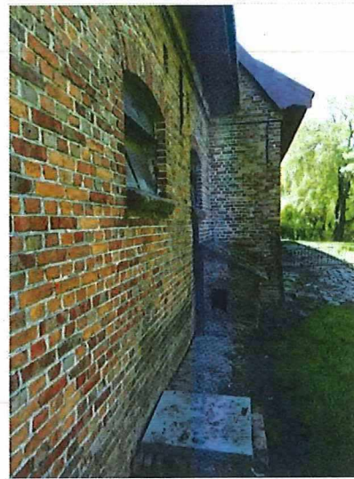
Foto 13: achtergevel met restant van de bakstenen verharding, stalvensters met bakstenen vensterbanken en hondenhok.
