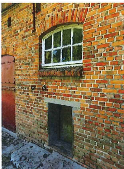
Foto 14: voorgevel met stalvenster, mestputopening en restant van de bakstenen verharding. Bovenaan zijn twee verluchtigsgaten van de stallen zichtbaar.
