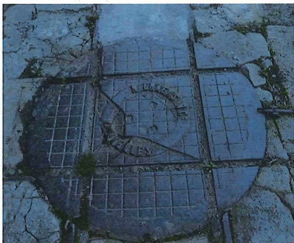
Foto 28: smalspoor voor de stallen - wissel of draaicirkel voor voeder- en machinekamer (met breuk) - opschrift "R. Eraers & Co, Bruxelles" (19.04.2018).
