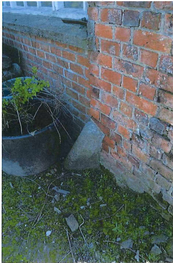
Foto 35: zij- of eindgevel van het koets- en wagenhuis - deels dichtgemetselde korbboogpoort - het schouderstuk van de tuitgevel zet aan boven de steunbeer (19.04.2018).
