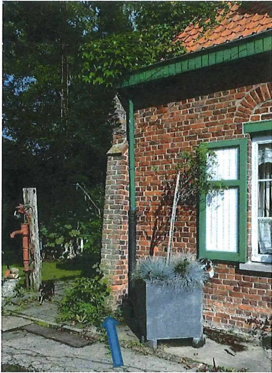
Foto 17: steunbeer op de hoek van de eindgevel en de langse gevel van de herenwoning – schouderstuk van de tuitgevel (30.08.2018).
