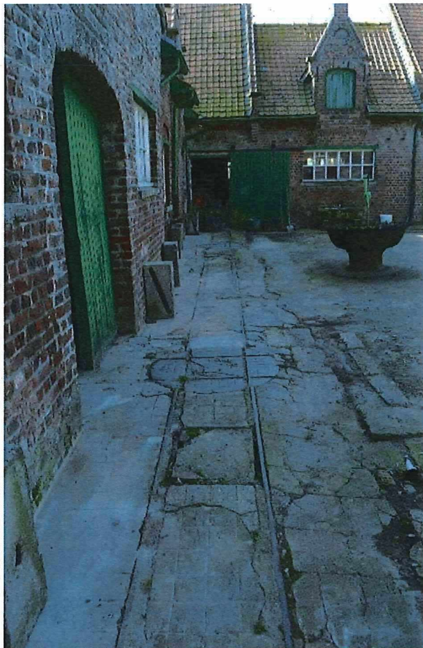
Foto 26: volume van voeder- en machinekamer met korfboogpoort, geflankeerd door stalvensters onder houten latei en korfbogige ontlastingsboog (19.04.2018).
