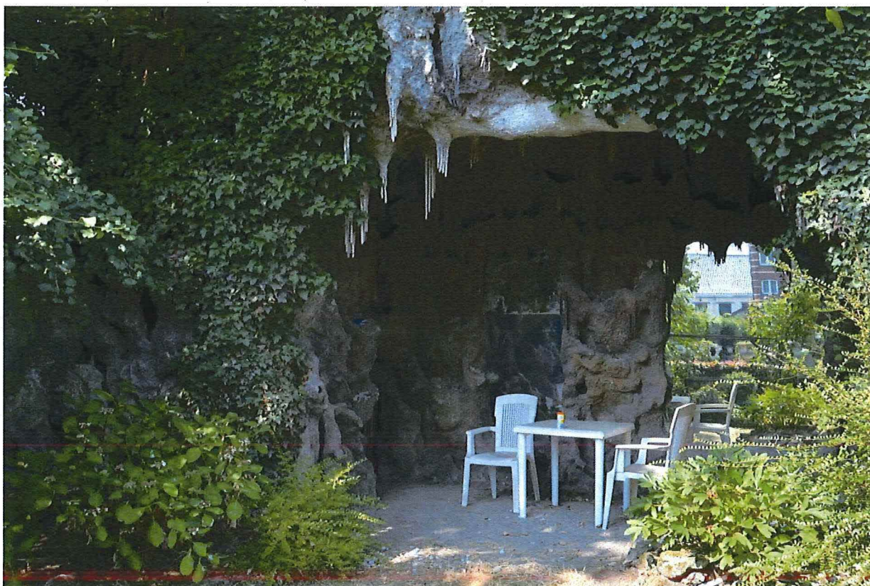
Foto 13: Mariagrot, met spiegels en stalactieten.
