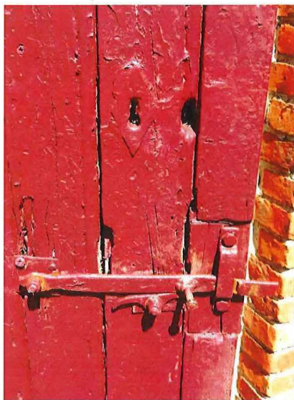
Foto 36: oorspronkelijke sleutelplaat en hang- en sluitwerk van de deur op foto 35.
