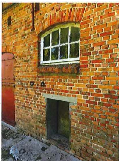
Foto 14: voorgevel met stalvenster, mestputopening en restant van de bakstenen verharding. Bovenaan zijn twee verluchtingsgaten van de stallen zichtbaar.
