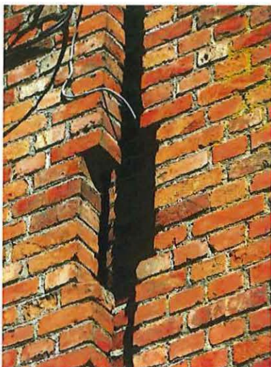
Foto 11: verluchtingspleet in de zuidelijke dwarsgevel.
