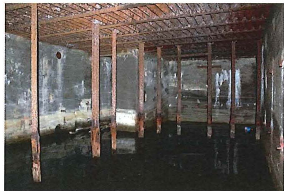
Foto 79: Bunker 40 (type VII). IJzeren structuur in bunker. Foto genomen door Tom Oliviers op 16 september 2016.
