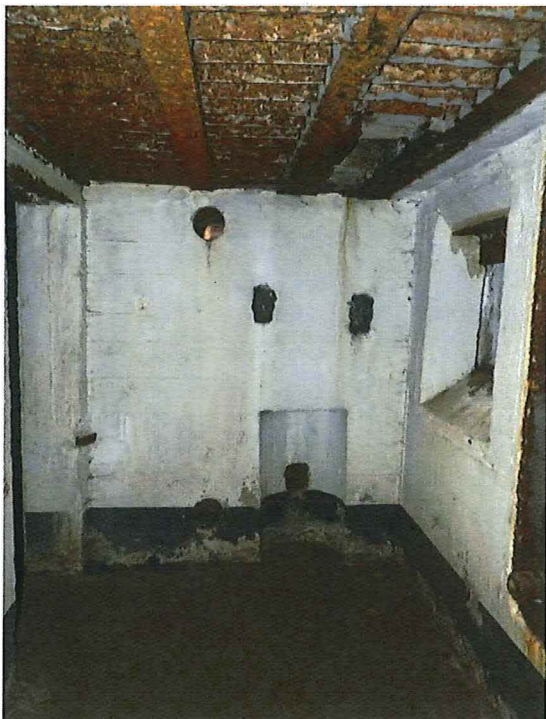
Foto 129: Bunker 60 (type VIII): interieur. Foto genomen op 21 februari 2018.
