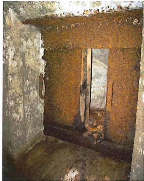
Foto 120: Bunker 57 (type VIII): Bewaarde schuiven vóór kijkgat. Foto genomen door Tom Oliviers op 17 juli 2013.
