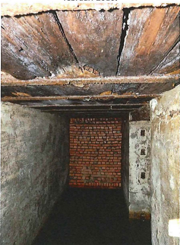
Foto 113: Bunker 54 (type II): gang achterzijde. Foto genomen op 21 februari 2018.
