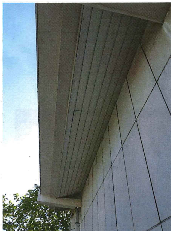
Foto 10: Gladbekist betonnen gootelement
