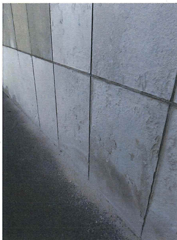
Foto 14: Lokale oppervlakkige aantasting portlandsteen.
