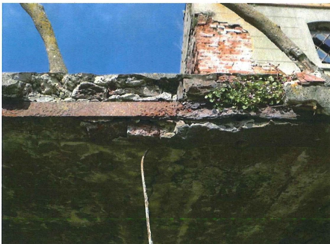
Foto 20: Detail van de wapening van het betonnen platform (© Bressers Architecten 22/11/2017).
