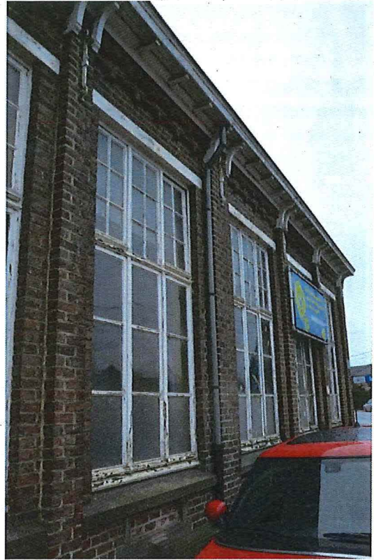
Foto 9: Detail raampartijen voorgevel. Ter hoogte van de lisenen bevinden zich de consoles van de dakoversteek (13/12/2017).
