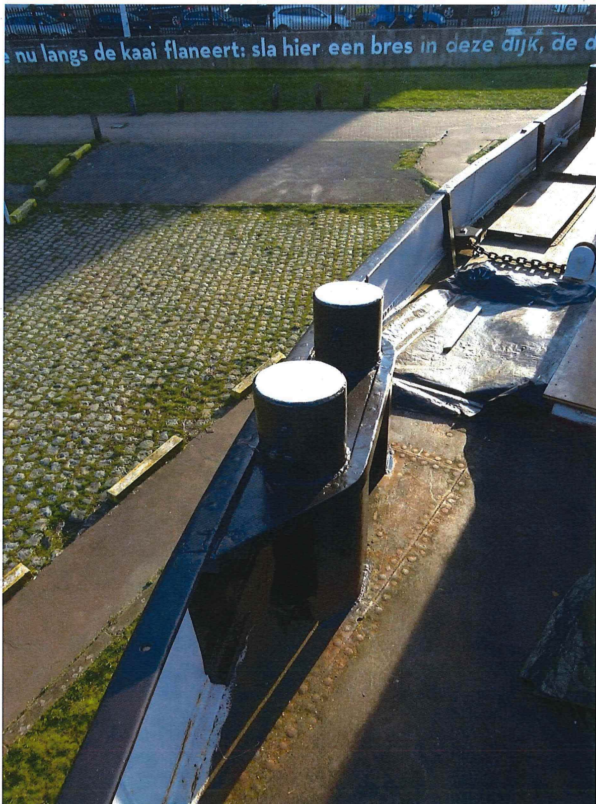
Foto 14: De dubbele bolder aan stuurboordzijde op het voordek.
