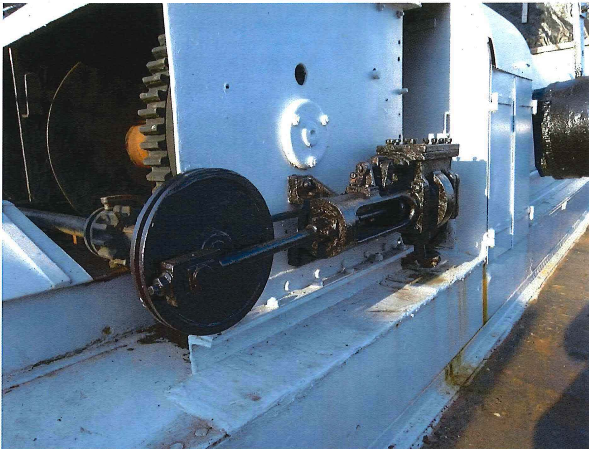
Foto 26: De lier wordt aangedreven door twee stoommachines, eentje aan iedere zijde van de lier. Gezicht op de stuurboordmachine.
