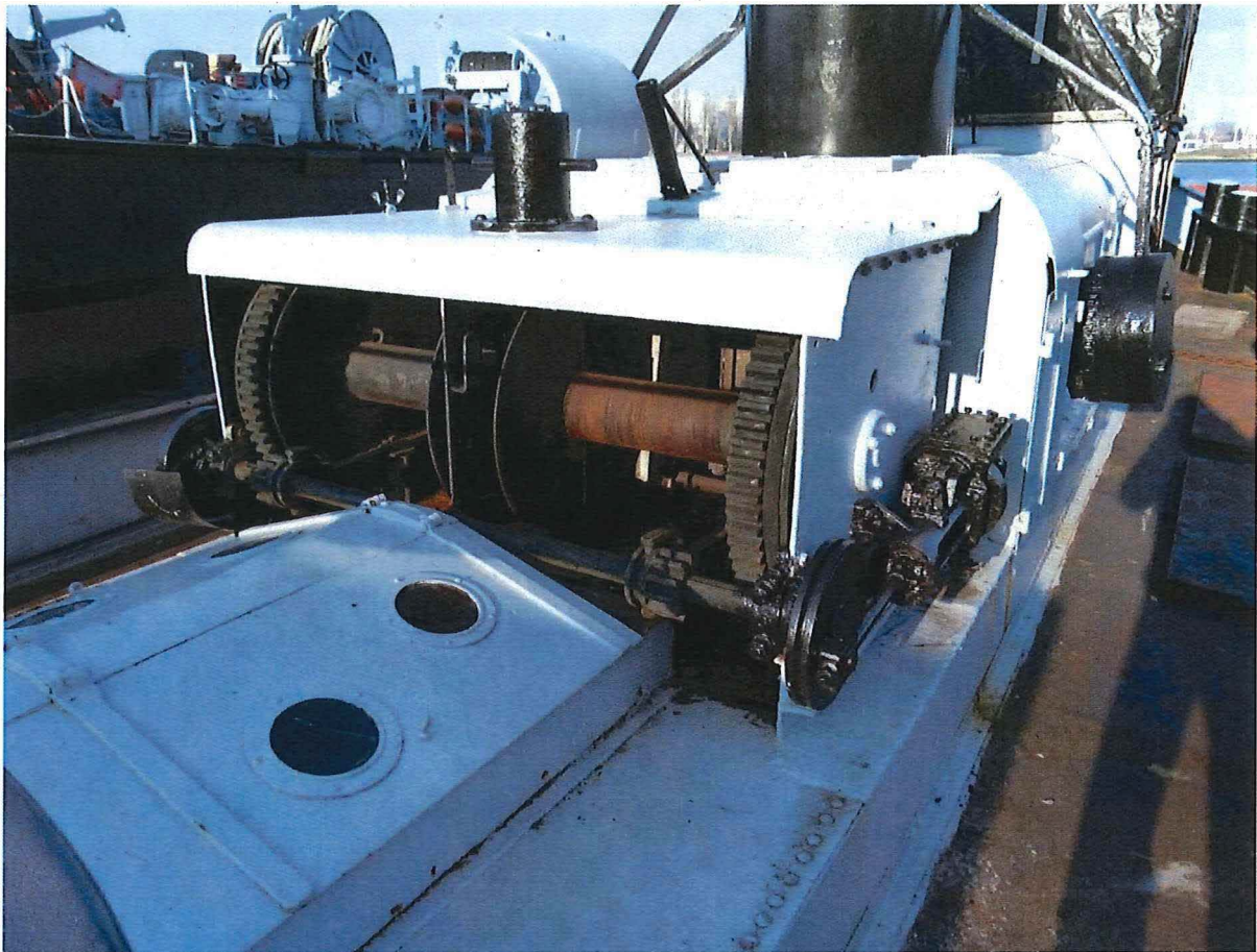
Foto 25: De lier met bolder staat op de vroegere plaats van de sleepbeting.
