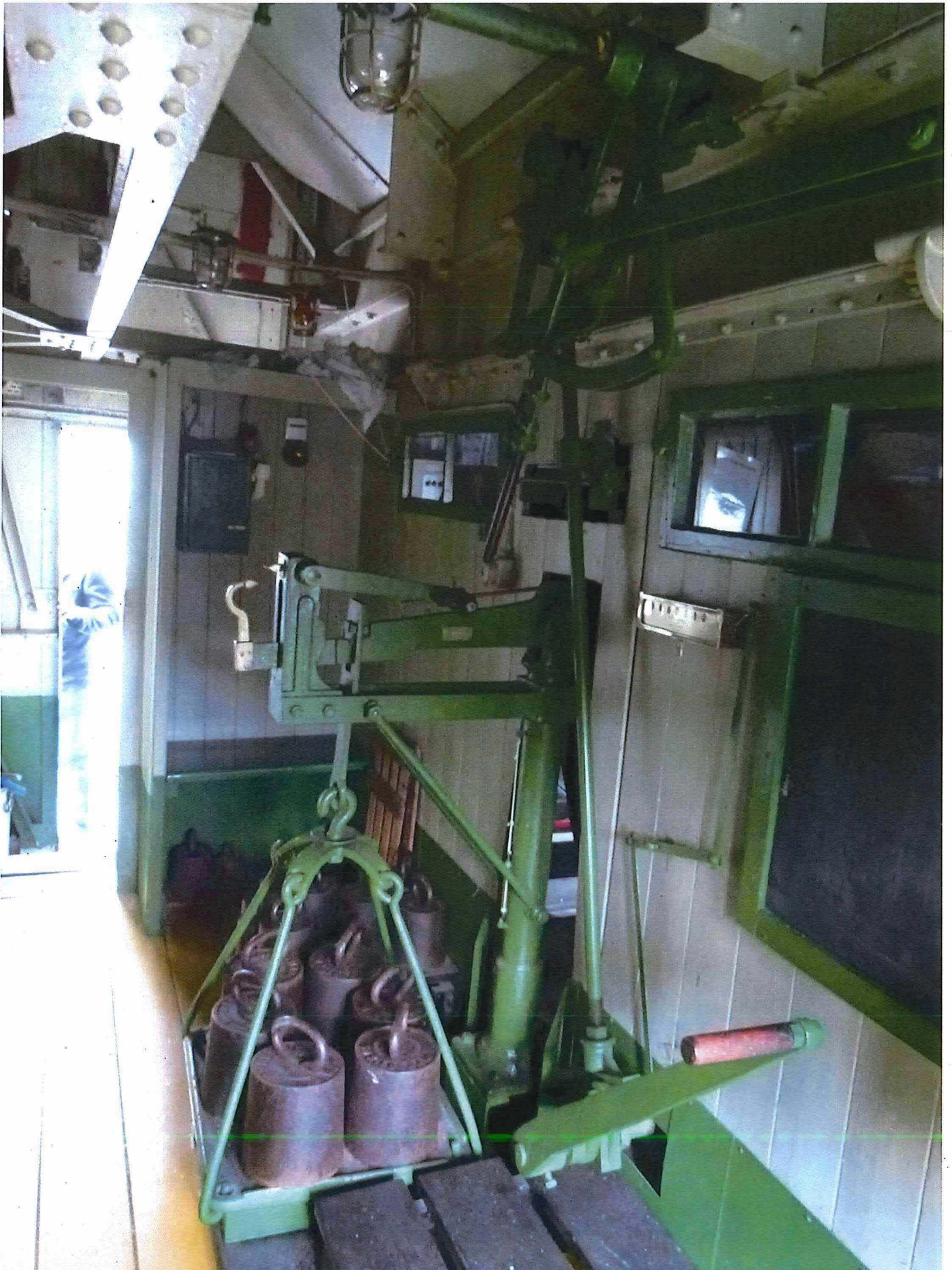
Foto 15: Kamer voor de bediening van de weegschaal en de schuif van de weegbak.
