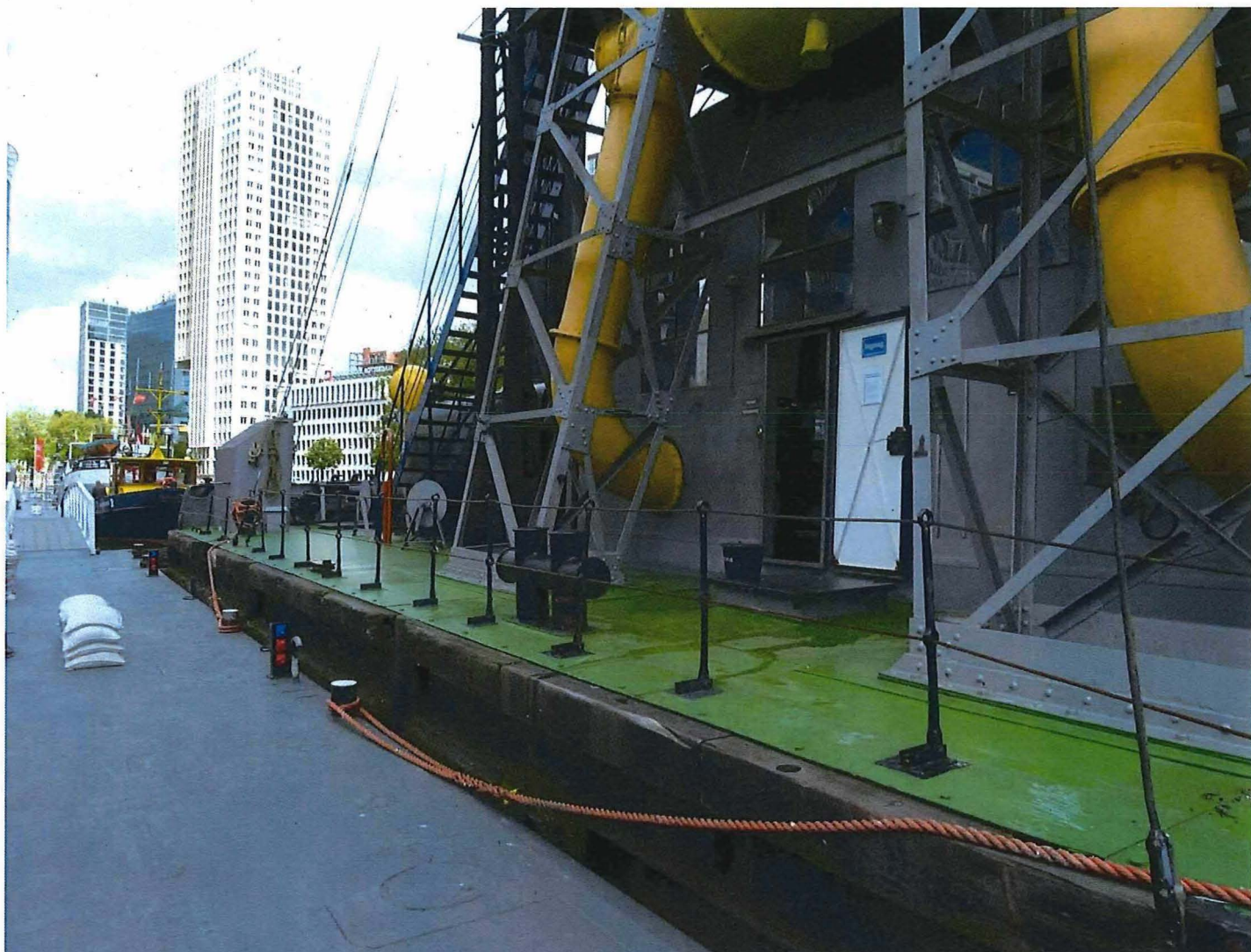
Foto 31: Zicht op de bakboordzijde van het vaartuig, met de toegang tot de machinekamer vanop het dek. De basis van de toren in stalen vakwerk is hier zichtbaar, evenals de twee luchtafvoerbuizen van de vacuümpompen.
