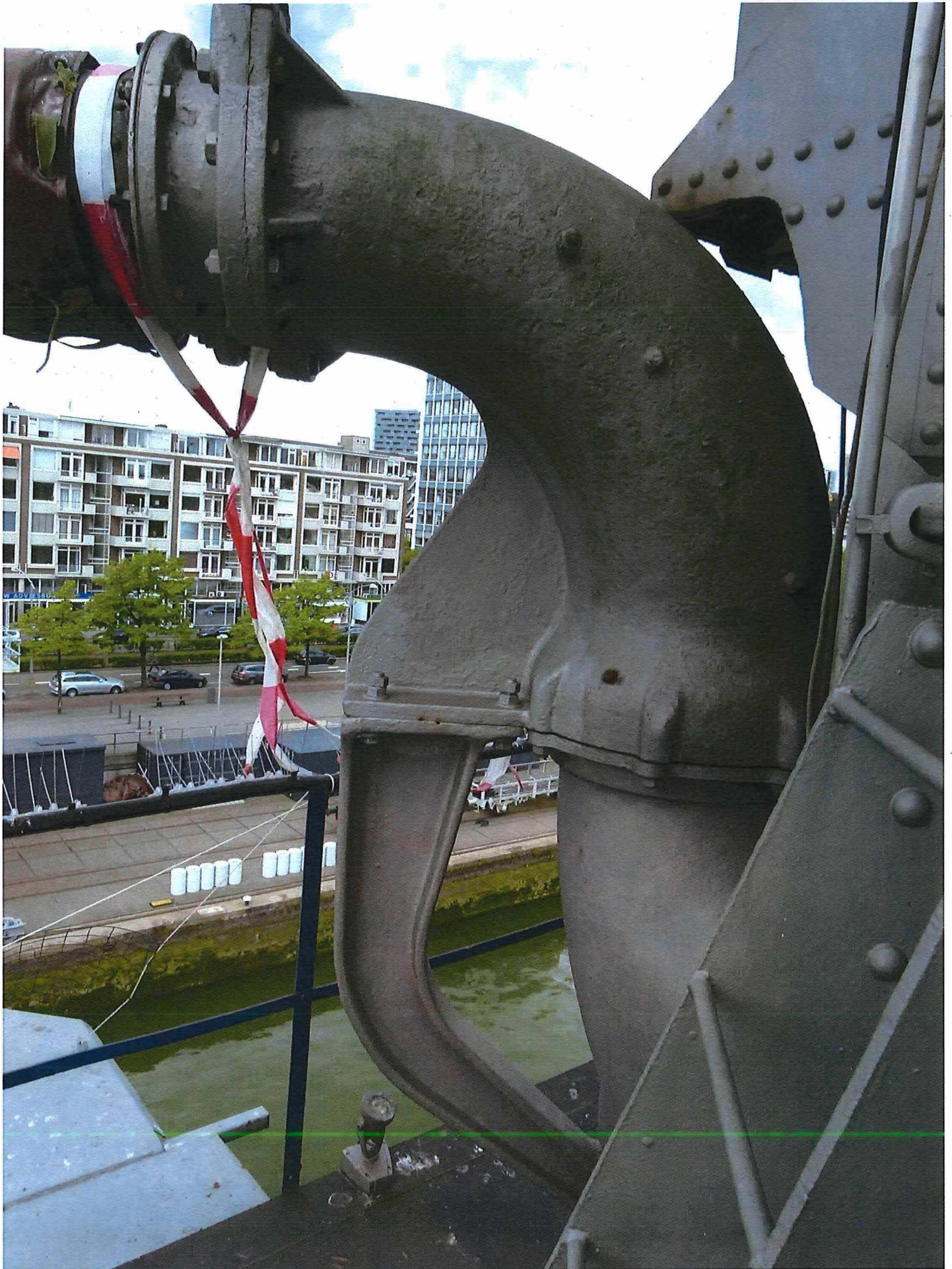
Foto 18: De aansluiting van één van de vier graanzuigleidingen op de recipiënt.
