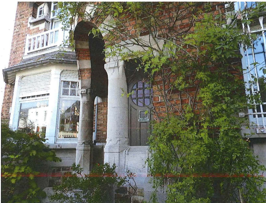
Foto 7: Zicht op het hoekportaal en het volume van het bow-window met balkon en borstwerking, gezien vanuit het zuidwesten (28/08/2017).
