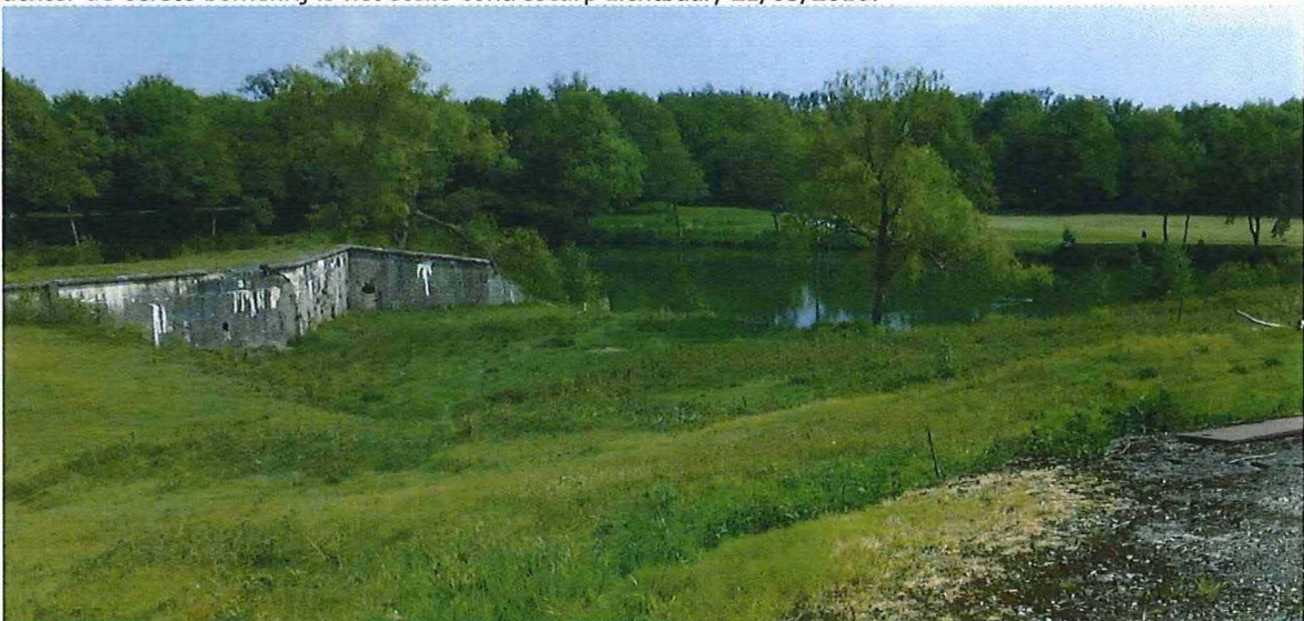
44. Caponnière met schietgaten, gaten voor 5,7cm snelvuurkanonnen en oreillon (schuinaflopemd). Centraal op de voorgrond bevindt zich de aangeaarde ondergrondse galerij naar de caponnière. In de achtergrond, achter de eerste bomenrij is het steile contrescarp zichtbaar, 21/05/2016.
