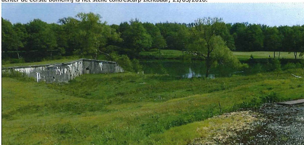
44. Caponnière met schietgaten, gaten voor 5,7cm snelvuurkanonnen en oreillon (schuinaflopnd). Centraal op de voorgrond bevindt zich de aangeaarde ondergrondse galerij naar de caponnière. In de achtergrond, achter de eerste bomenrij is het steile contrescarp zichtbaar, 21/05/2016.
