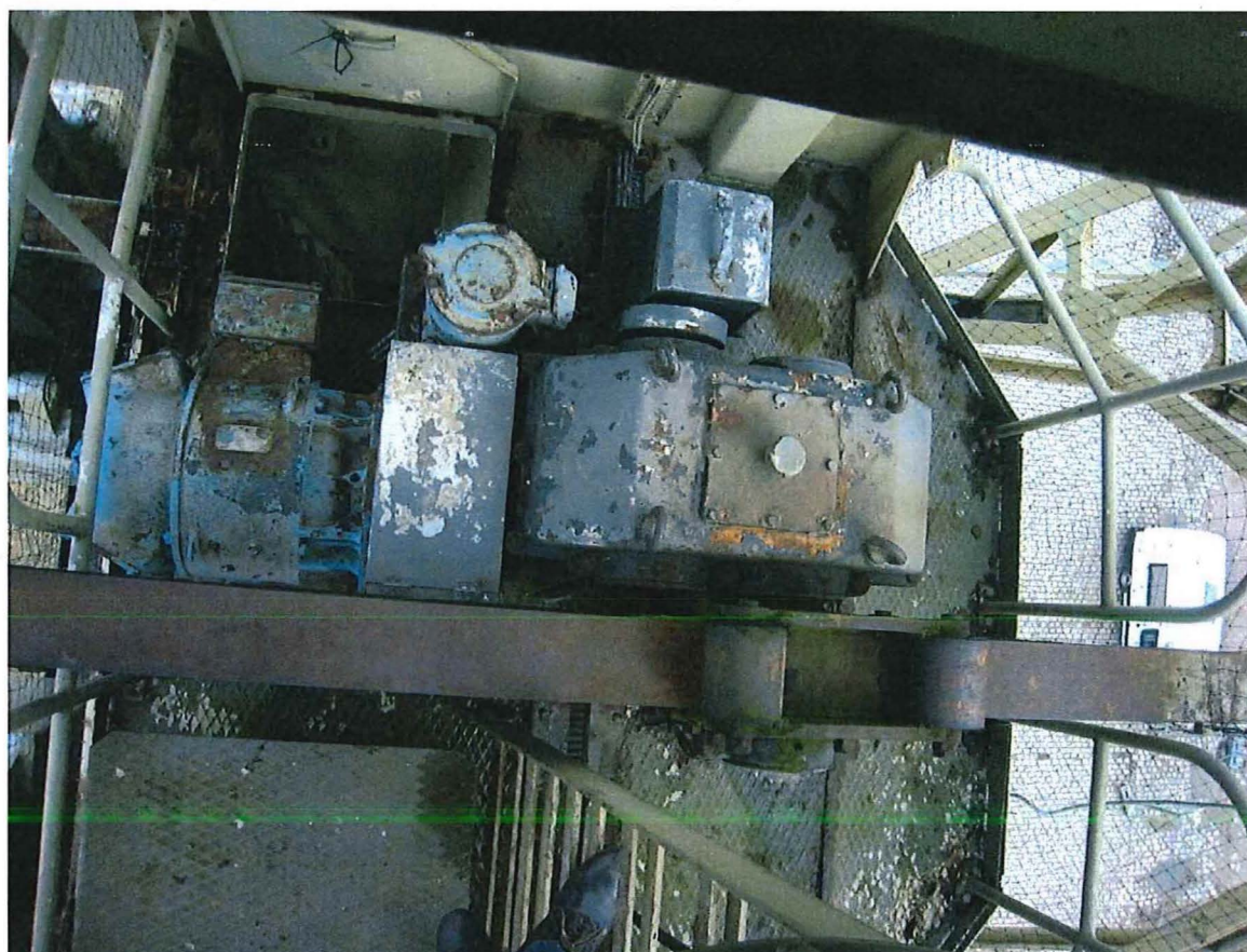
Foto's 31 en 32: Op het tweede niveau staat de topinstallatie van de kraan. Die bestaat uit een elektromotor die via een overbrenging een rondsel aandrijft en zo de tandheugel vooruit of achteruit beweegt. De leidrollen van de heugelstang zijn bovenop zichtbaar.
