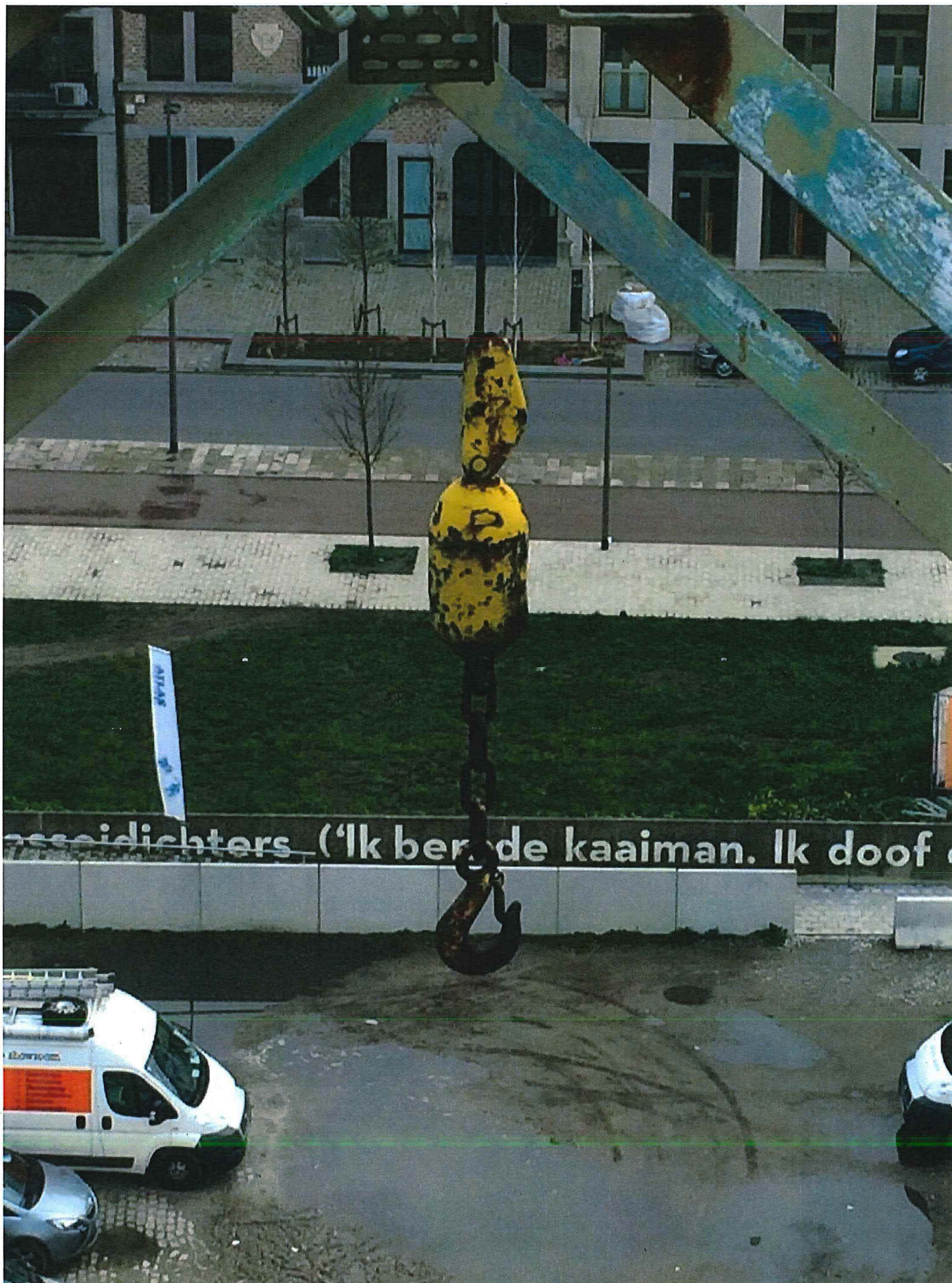
Foto 42: De hijshaak.
