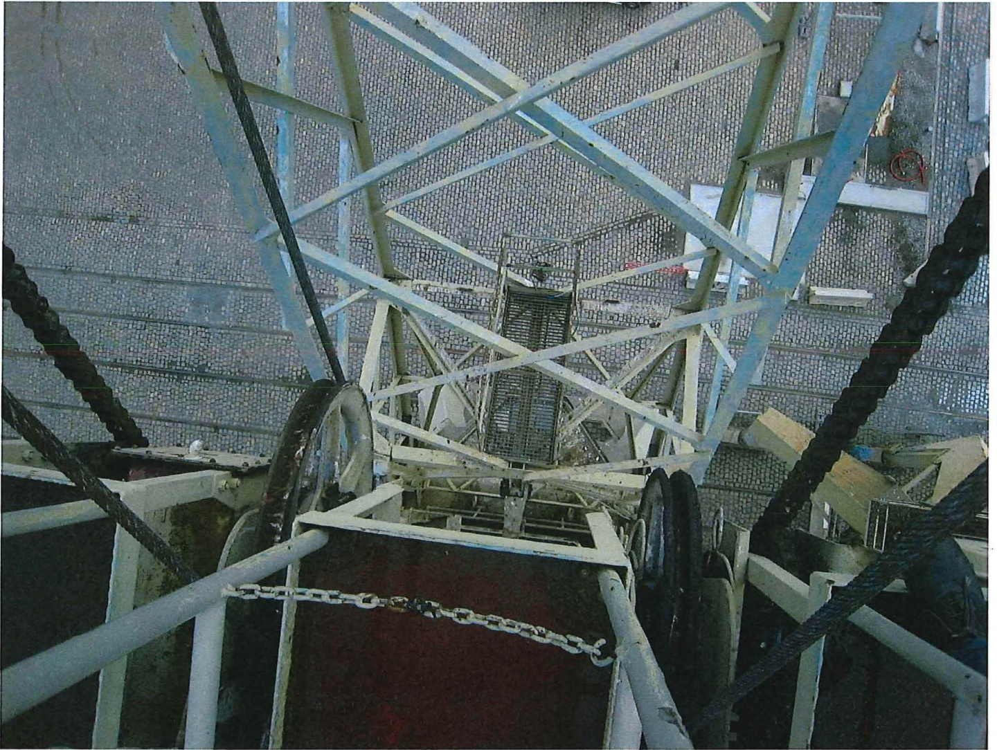
Foto 39: Vanop het platform aan de zijde van de giek zijn de twee volgende kettingwielen zichtbaar voor de geleiding van de ketting van het tegengewicht. De twee schijven zorgen voor de geleiding van de hijskabel. Rechts op de foto loopt de hijskabel van de trommel naar de top van de giek om daar via een keerschijf terug te lopen naar de keerschijf links op de foto. Die schijf geleidt de kabel naar de top van de giek.
