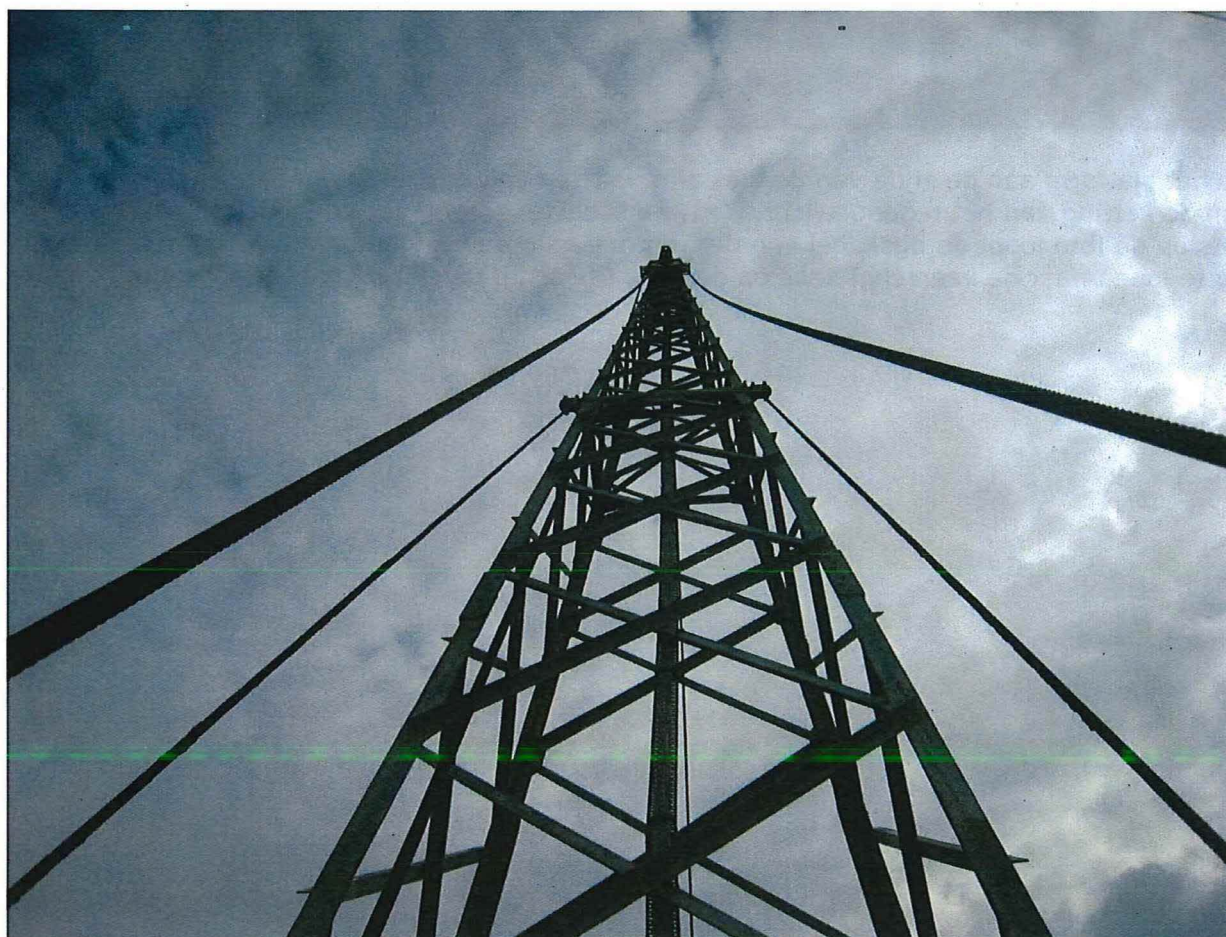
Foto's 40 en 41: De schakels die de kettingen van het tegengewicht verbinden met de ophangkabels (foto boven). De giek in vakwerk met de bevestiging van de kabels van het tegengewicht en in de giekkop de keerschijf voor de hijskabel (foto onder).
