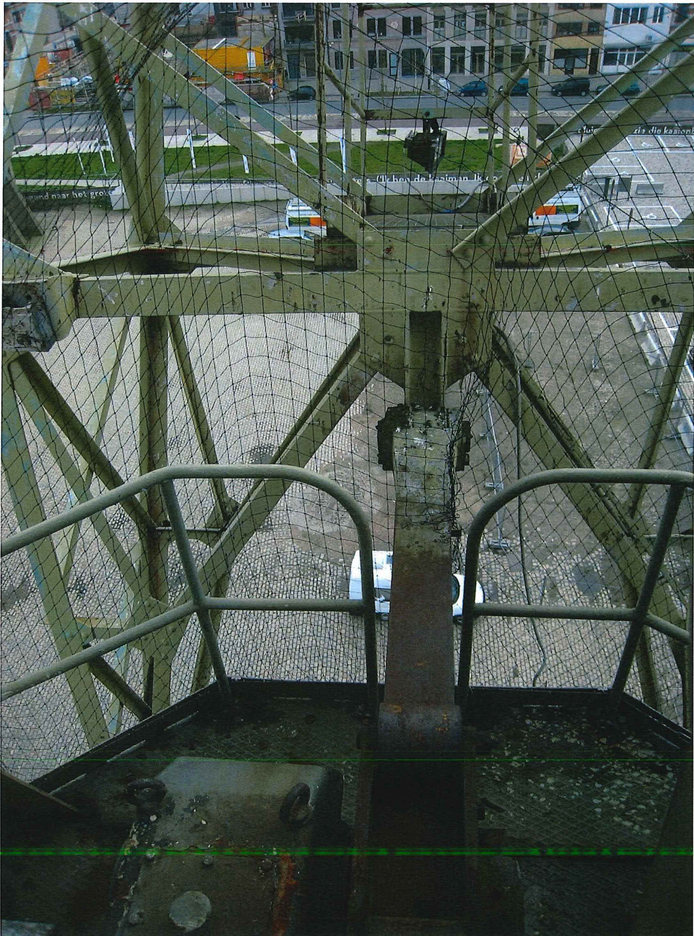
Foto 33: De heugelstang is verbonden met de giek en kan de giek verder weg van de toren laten zakken of de giek naar de toren toe trekken (toppen).
