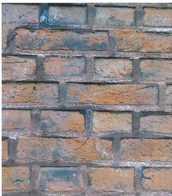
Foto 9-10: Nijverheidsschool (1857-1859) voorgevel: gekleurde knipvoegen en friezen met verluchtingsrooster
