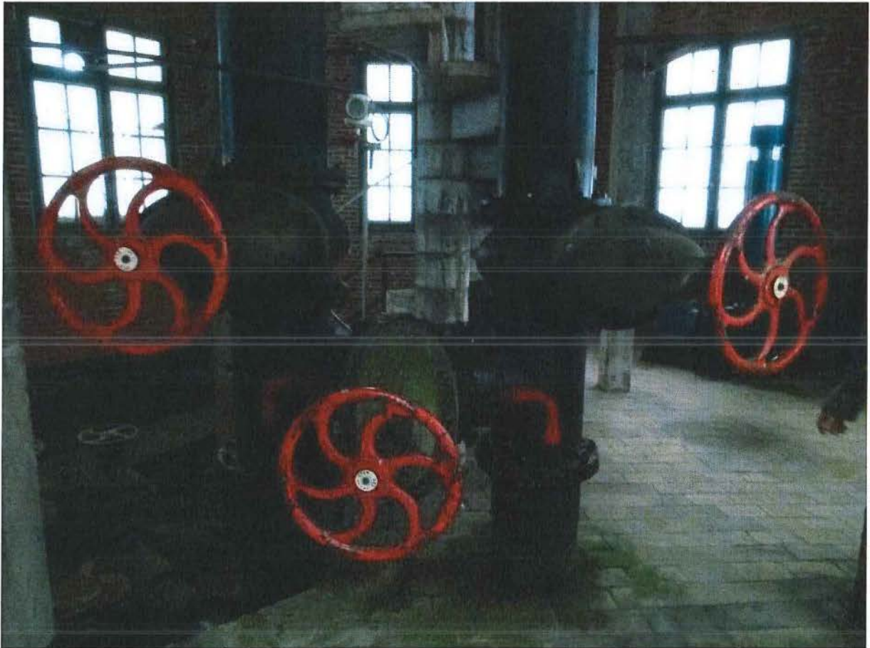
Foto 7: De twee standleidingen voor aanvoer en distributie van het water, met de bypass.
