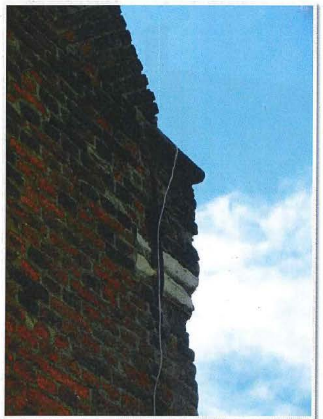
Foto 13: zuidelijk schouderstuk van de achtergevel van het voorhuis.
