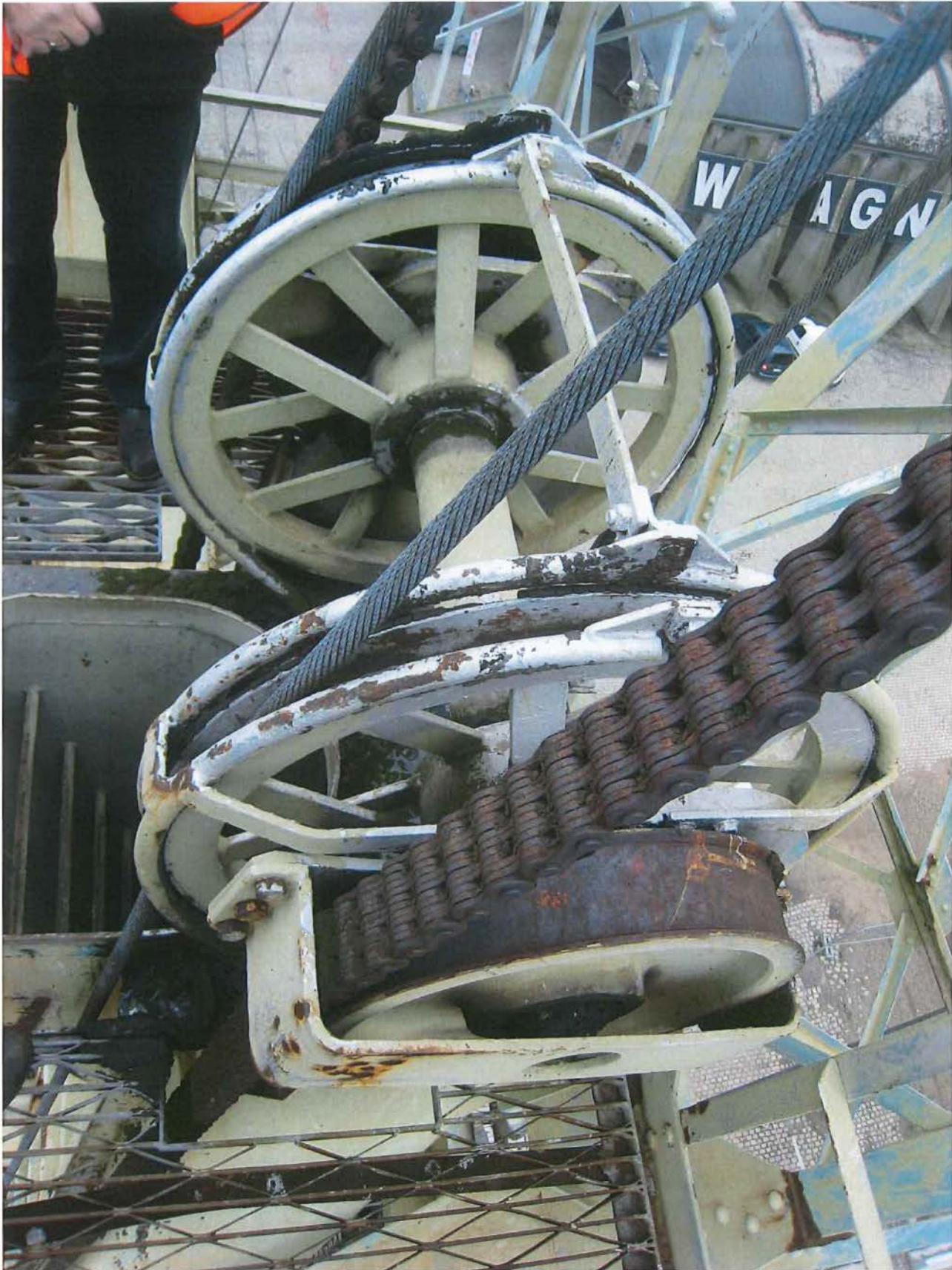
Foto 20: De top van de toren met de geleidingsschijven voor de fleyerkettingen die het tegengewicht aan de giek bevestigen en de kabelschijven van het hijsmechanisme.
