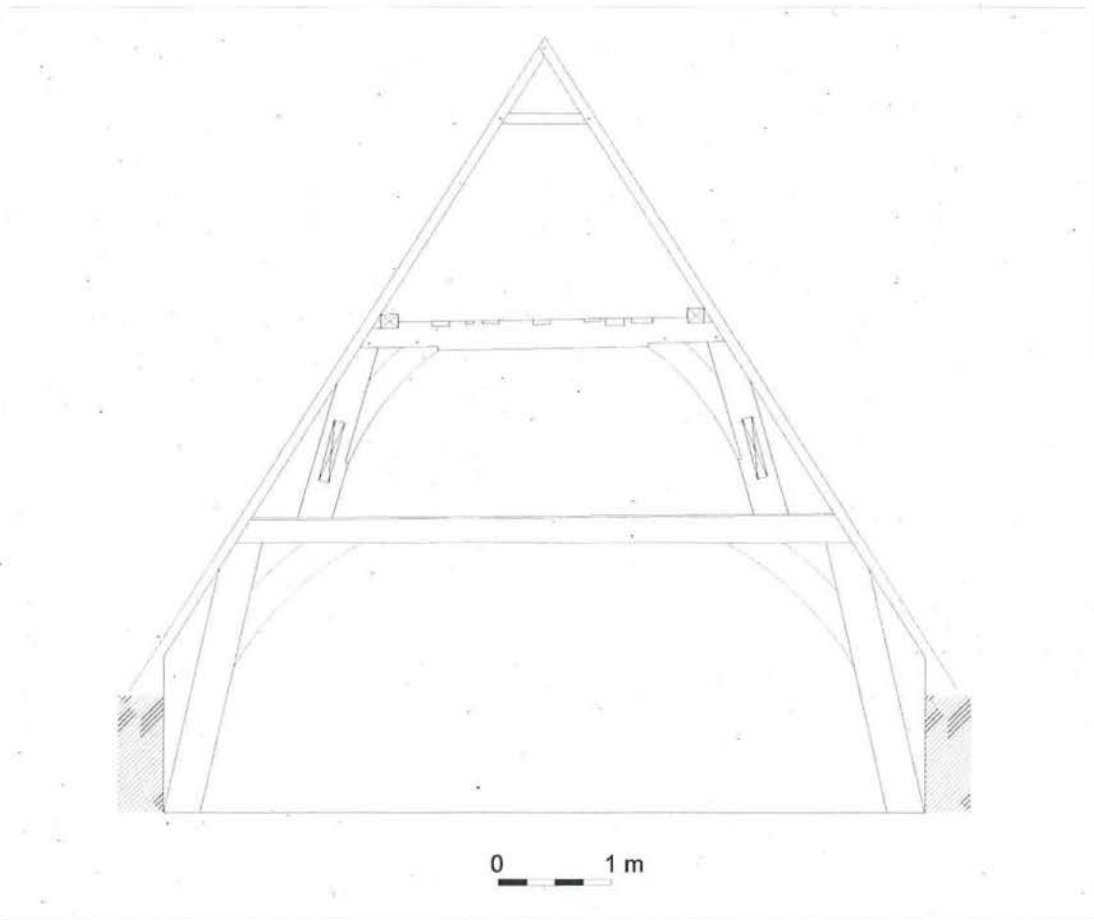
Foto 6: opstand van de dakkap, met suggestie van het onderste, thans niet zichtbare schaargebint. De constructie van de voeten van de sporen kon niet worden vastgesteld.
